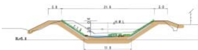
筋生野橋付近標準断面図
