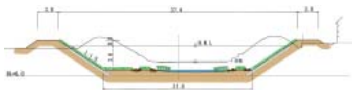
豊橋付近標準断面図
